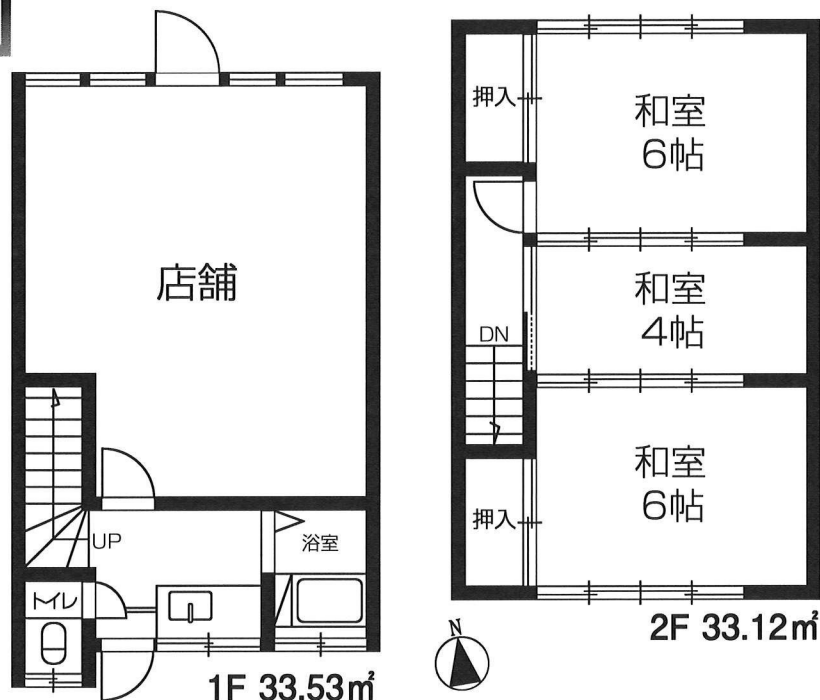
【配置図】
