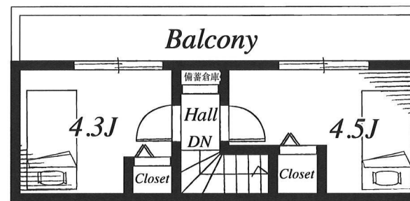
3F 19.05m²
