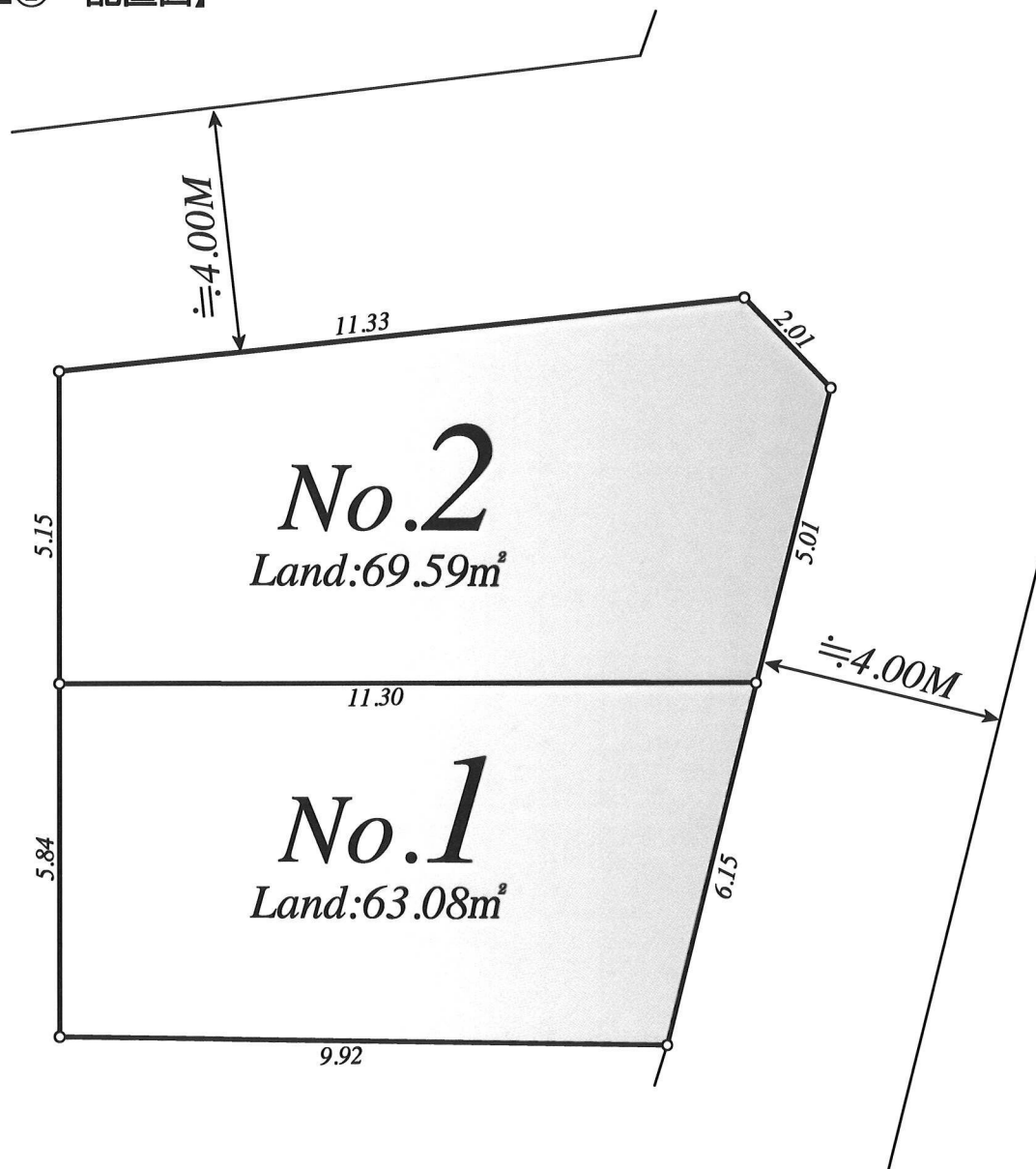
【国分寺市東恋ヶ窪302② 配置図】
