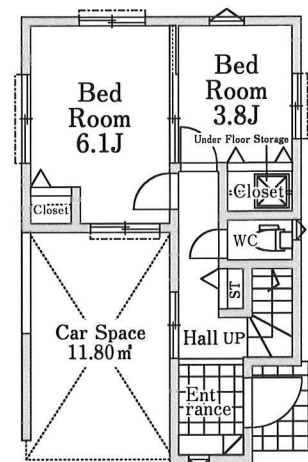
1F 39.33㎡(車庫面積11.80㎡含む)
