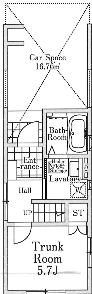
1F 39.27㎡ (車庫面積16.76㎡含む)
