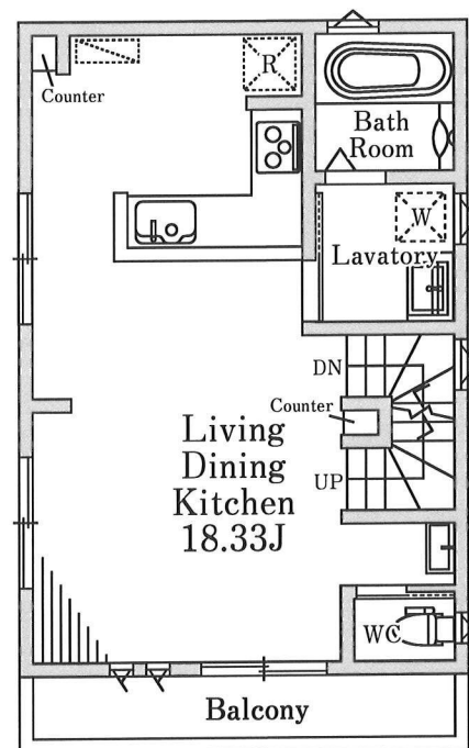
2F 43.99㎡
